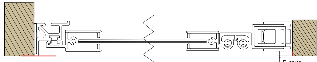
In de dag montage Zij-aanslag
